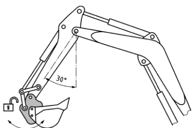
Abbildung: Prüfung Haltefunktion (Quelle: EN 474-5 : 2022)
